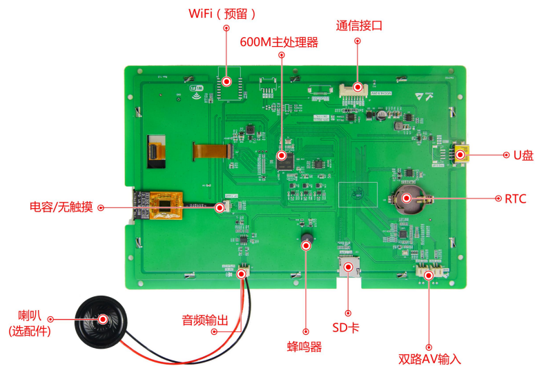
图 1-3 硬件配置图
